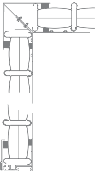
파사드 코너 상세도
