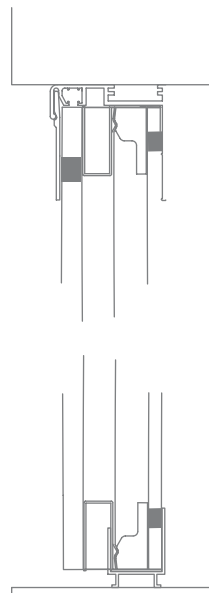
파사드 상하부 상세도
